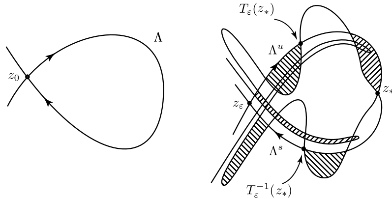
Рис. 23.6: Сложное поведение сепаратрис при \varepsilon \neq 0 (справа) в отличие от невозмущенного случая (слева) на сечении Пуанкаре \{(x, y, t) : t = 0 \bmod 2\pi\} . Заштрихованные области (лунки) переходят друг в друга при отображении T_\varepsilon . Поэтому их площади равны.
