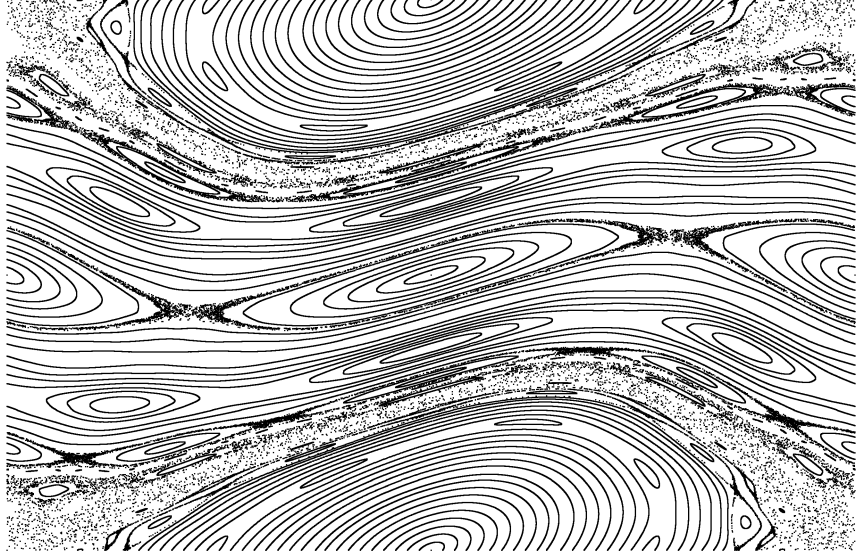
Рис. 22.5: Траектории стандартного отображения при \varepsilon = 0.14 . По сравнению с рис. 22.4 хаотические облака более заметны.
