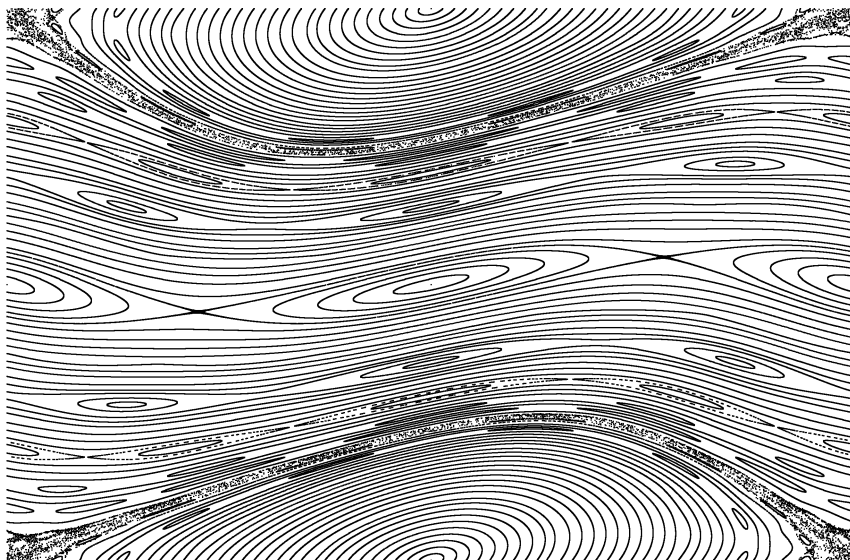
Рис. 22.4: Около сотни траекторий стандартного отображения при \varepsilon = 0.9
