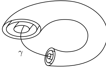
Рис. 21.3: Инвариантные торы, окружающие кривую \gamma на M_h .
