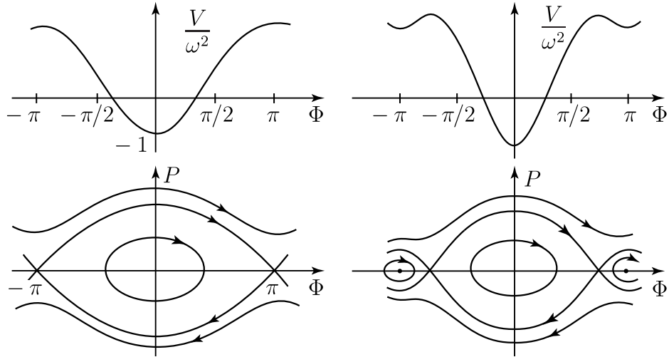
Рис. 10.1: Фазовые портреты: слева при a^2 < 2l^2 , справа — при a^2 > 2l^2 .
