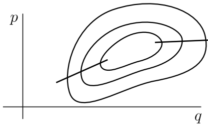
Рис. 15.2: Линии уровня функции H(q, p) (они же — кривые \gamma_h ). На двух "горизонтальных" кривых \partial H / \partial p = 0 .
